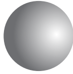
X küresi
